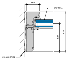
⑦ JAMB AT FIXED LITE 6\"/>
