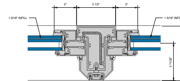
⑨ FIXED MULLION D' = 1'-0"
