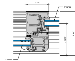
⑫ INTERLOCK 6\"/>
