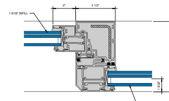
⑨ INTERLOCK 6\"/>
