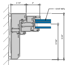
⑦ JAMB AT FIXED LITE 6\"/>
