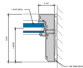
⑨ JAMB AT FIXED LITE 6\"/>
