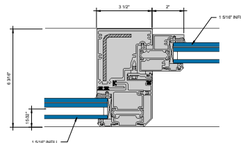
⑧ INTERLOCK 0\"/>
